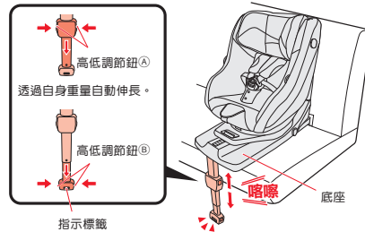
指示標籤
