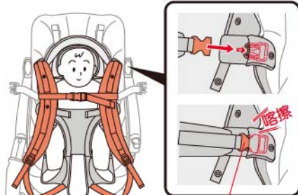
揹巾安全揹帶固定扣 (紅色)
